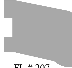
FL # 207 1-1/8"x 1-3/8"
